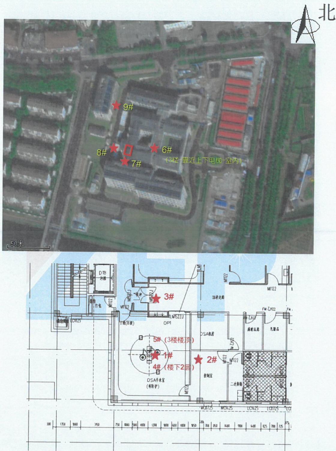
DSA 机房建设项目环境 \gamma 辐射剂量率监测点位示意图
