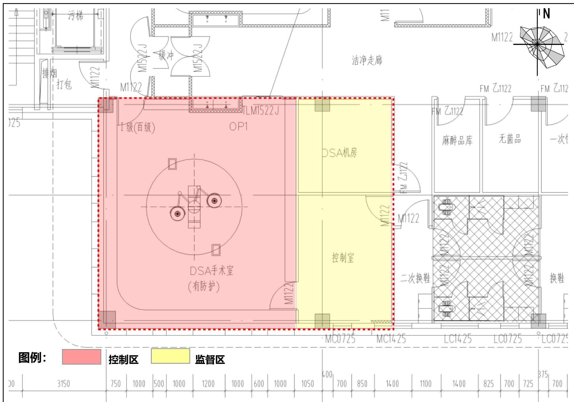
附图4 本项目辐射分区示意图
